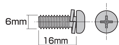
④スクリューA×4本(6×16mm)
