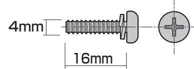
⑤スクリューB×2本(4×16mm)
