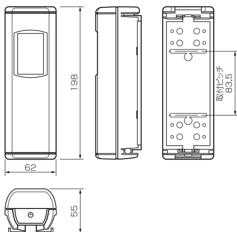
〈外形寸法図〉
