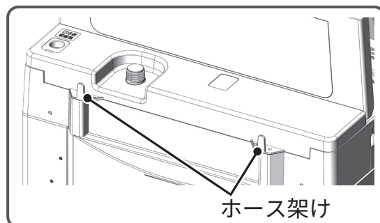
背面図
