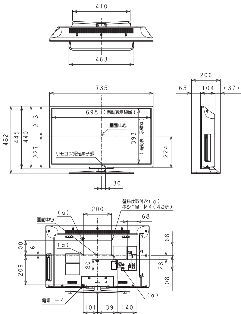
壁掛けユニット(別売)取り付け時の寸法
