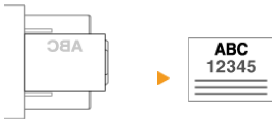
ヨコ向きの用紙（コピー時）
