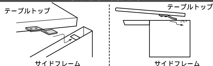
拡大図・側面図
