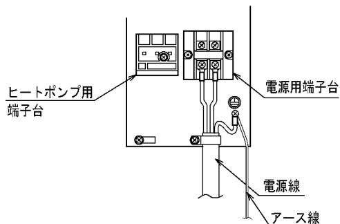
貯湯タンクユニット電気品取付板
