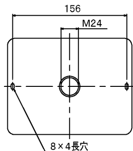
取付寸法図
