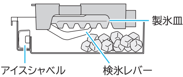
横から見た断面図
