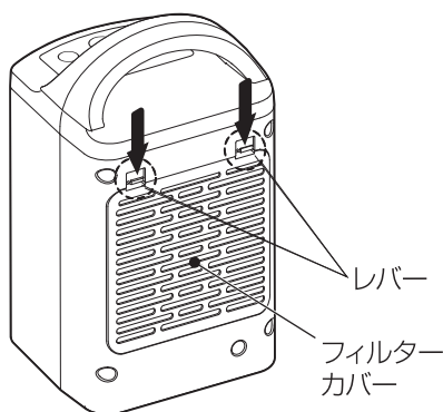
フィルターカバー上部の レバー2ヶ所を押し下げる
