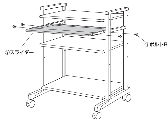
⑫ボルトB [M4×6]
