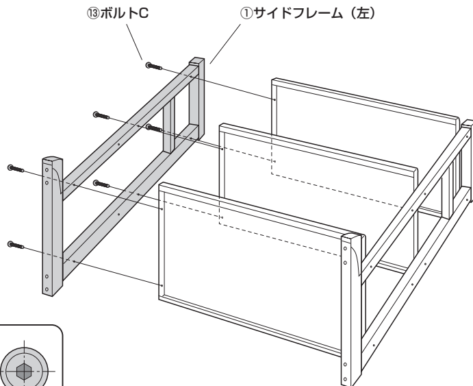
⑬ボルトC [1/4"×35]
