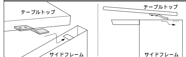
拡大図・側面図
