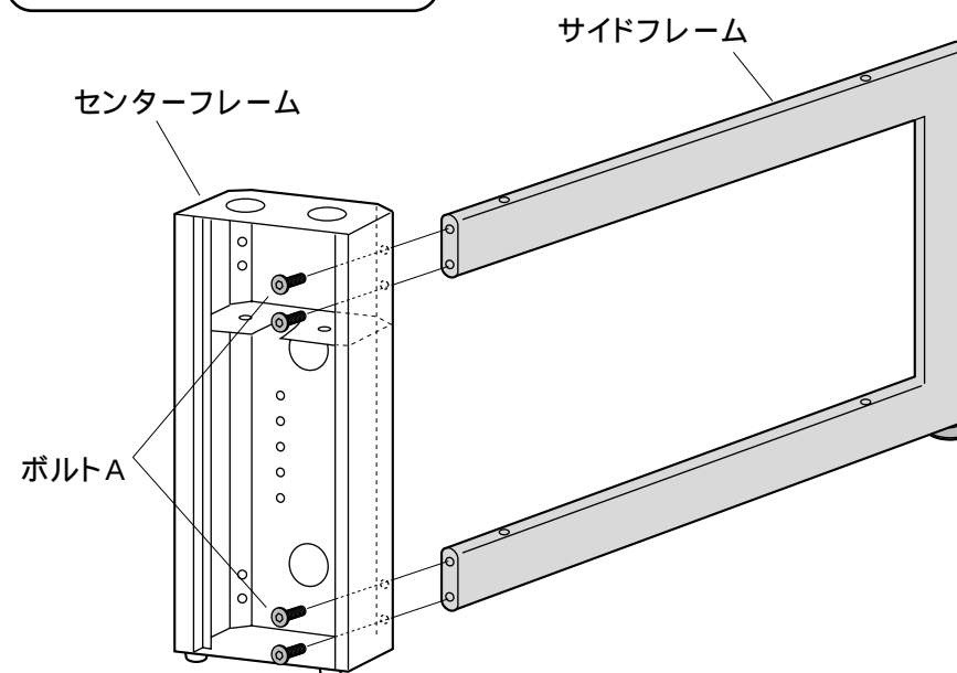
ボルトA [M6 × 20]
