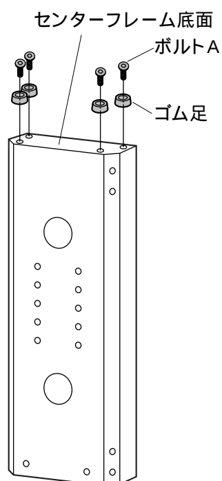
ボルトA [M6 × 20]
